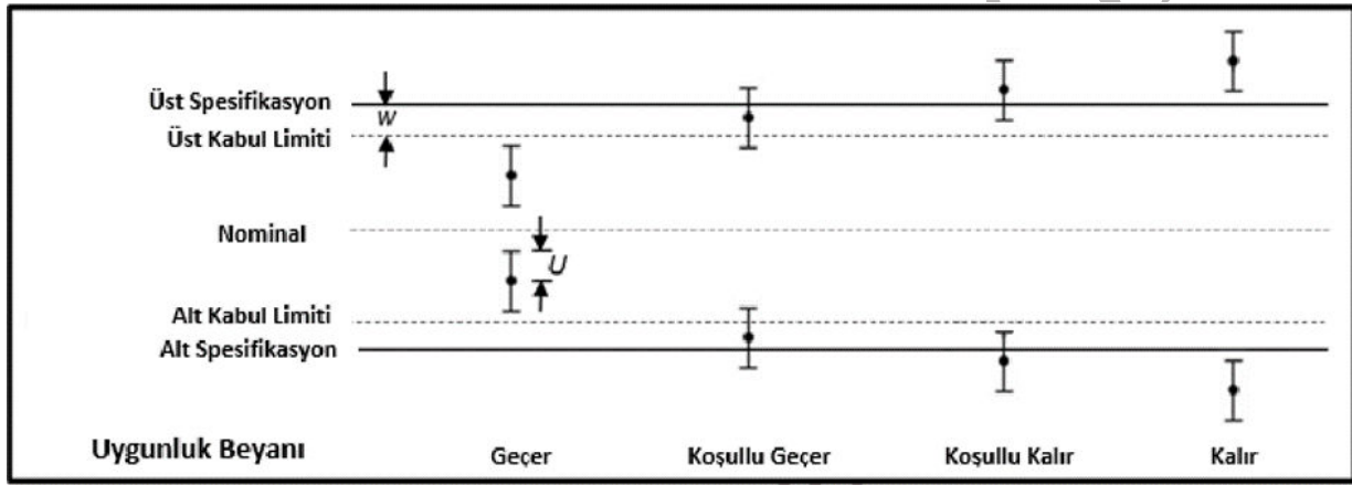
Şekil 4. Koruma Bantlı İkili Olmayan Beyanın Grafikselsel Gösterimi
